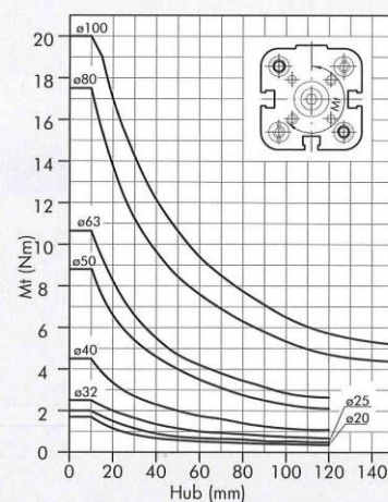
DREHMOMENT IN ABHÄNGIGKEIT VOM HUB
