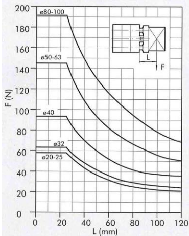
SEITENLAST VERDREHGESICHERT
